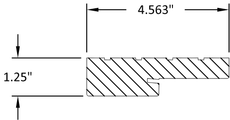
2 SIDELIGHT JAMB
