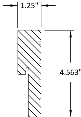
2 SIDELIGHT JAMB
