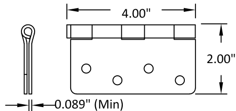
4 BUTT HINGE 12 GA. STEEL
