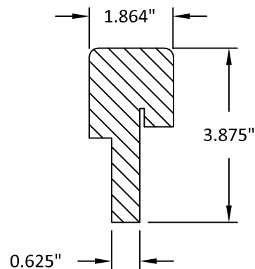
10 ASTRAGAL
